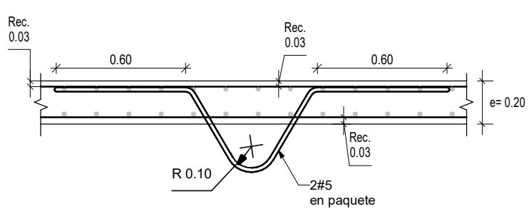
DETALLE GANCHO DE IZAJE ASCENSOR Escala 1 : 25
