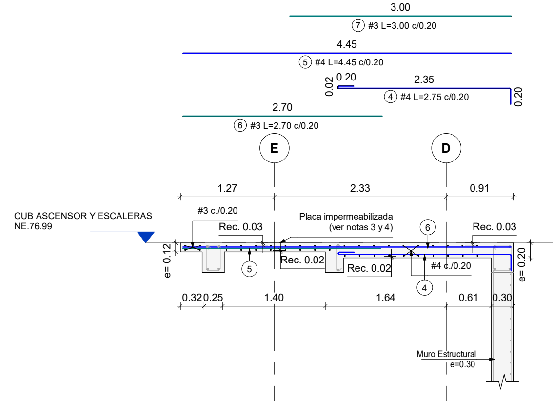
CORTE CM-3 Escala 1 : 50
