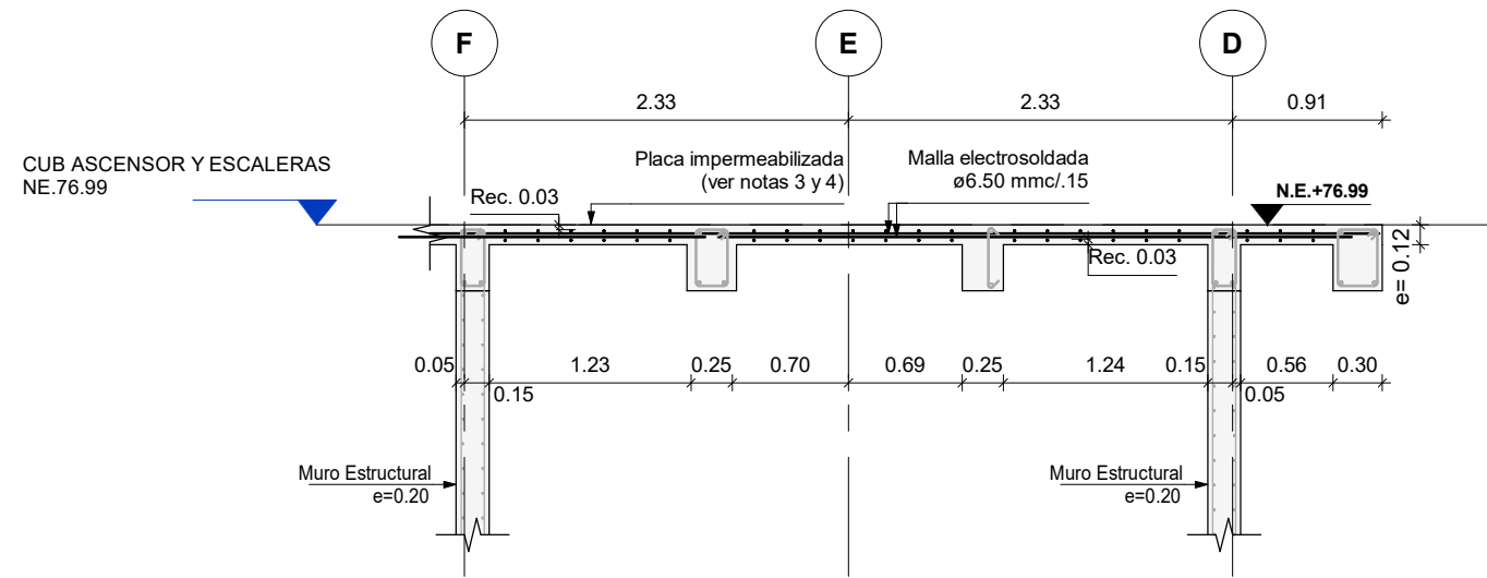
CORTE CM-2 Escala 1 : 50
