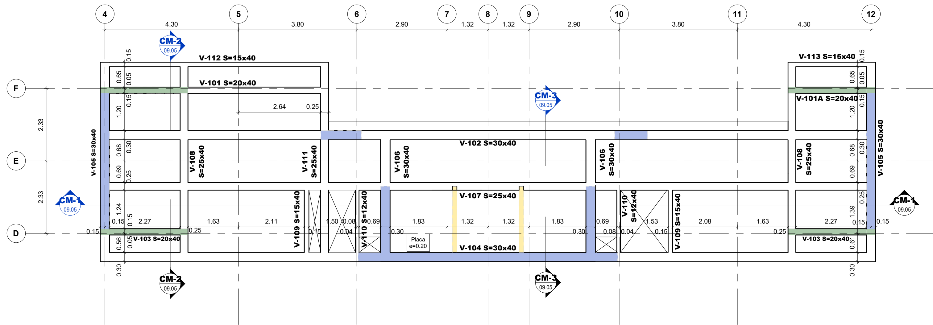
PLANTA CUBIERTA FOSO DE ASCENSOR Y DE ESCALERAS N.E. 76.75 Escala 1 : 75
